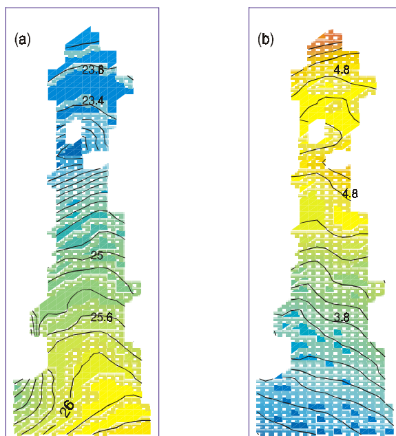
Figura 3. Distribución espacial del (a) promedio total de la temperatura superficial del mar y (b) su desviación estándar. El intervalo de contornos es 0.2°C.
