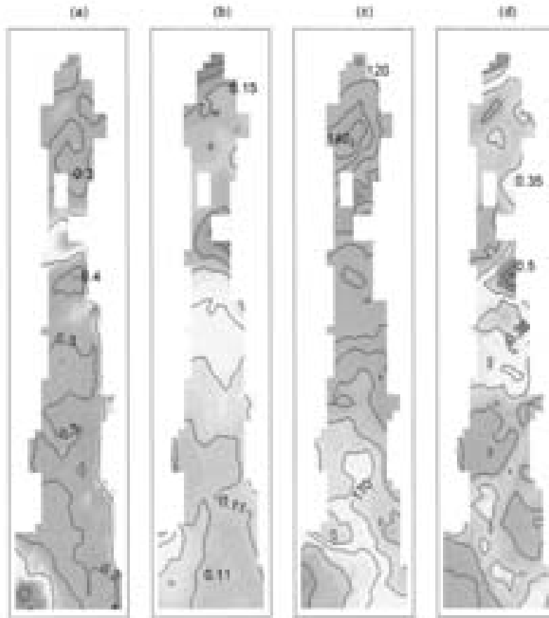
Figura 11. Distribución espacial de (a) la amplitud y (b) su error (°C), y de (c) la fase y (d) su error (meses), para la componente interanual de la temperatura superficial del Golfo de California. Figure 11. Spatial distribution of (a) amplitude and (b) its error (°C), and of (c) phase and (d) its error (months), for the interannual component of surface temperature of the Gulf of California.
