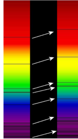
Espectro de absorción
